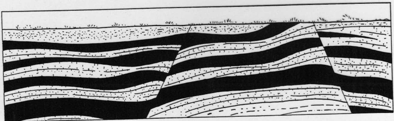
Abb. 8.23: Entstehung der Steinkohle nach einer typischen Schulbuchdarstellung. Sie illustriert in sehr vereinfachter Form die Theorie der autochthonen (am Fundort entstandenen) Bildung der Steinkohle. Am Rande sei bemerkt, daß in diesem skizzenhaften Entwurf die Flöze zu mächtig und die Zwischengesteine zu dünn eingezeichnet sind und der Inhalt des Torfes unrichtig dargestellt ist, vgl. Abschnitt 8.5.4. (Nach Bär 1977)
